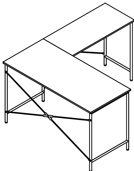
＜天板（小）を右側に取り付ける場合＞
